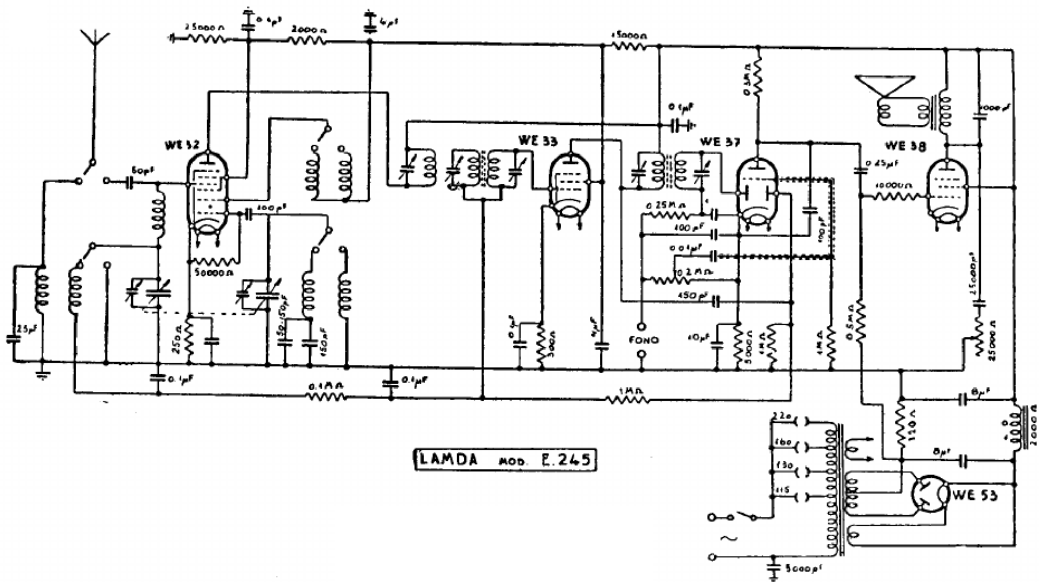
OLIVIERI e GLISENTI. — Modello Lamda E 245. — Produzione 1938-39. — Media frequenza: 467 kHz.
